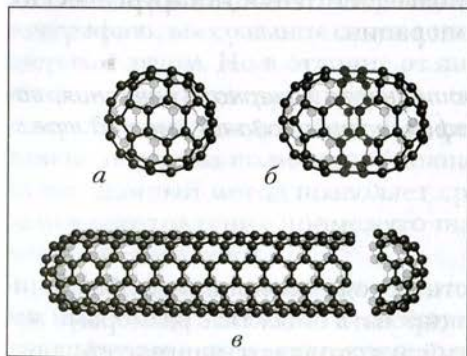
Рис. 20. Наномолекулы: а — фуллерен C_{60} ; б — удлинённый фуллерен C_{70} ; в — нанотрубка
